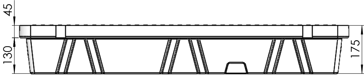
SEZIONE A-A SCALA 1 : 8
