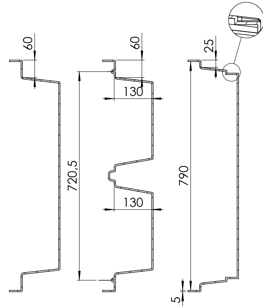
SEZIONE D-D SCALA 1 : 8
